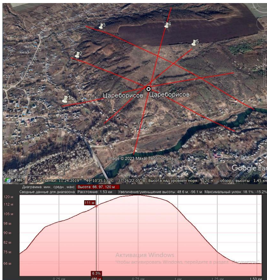
Рис. 5. Детализация рельефа посредством построения серии профилей в зоне предполагаемого расположения крепости
